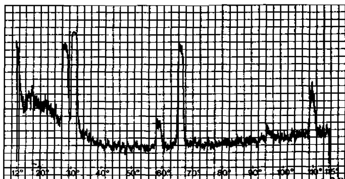
Fig. 15.9 NaCl 30 kV
